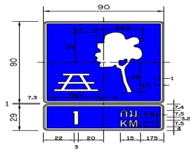
ป้ายแสดงที่พักริมทาง
