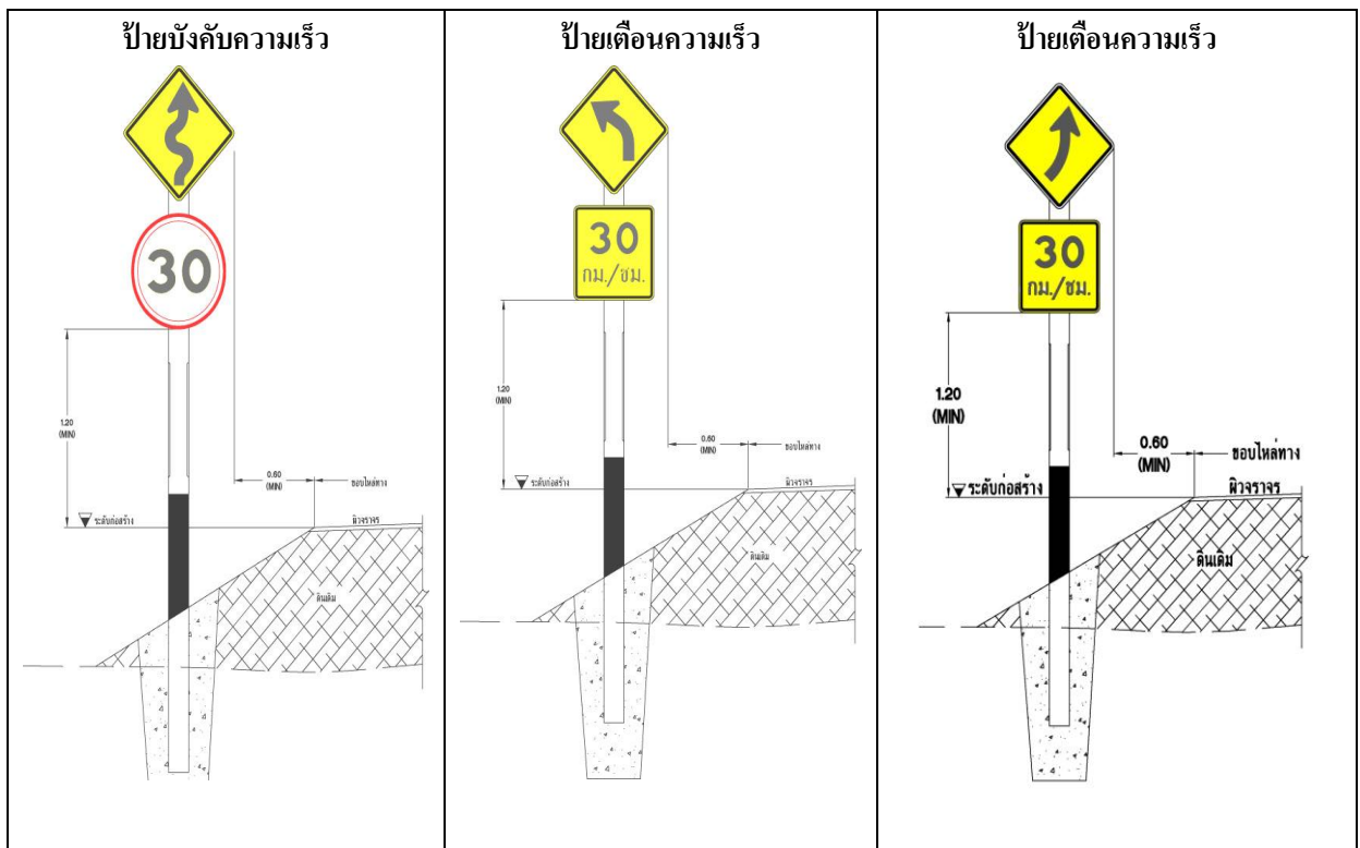
รูปแสดงมาตรฐานการติดตั้งป้ายชนิดเสาเดี่ยว
