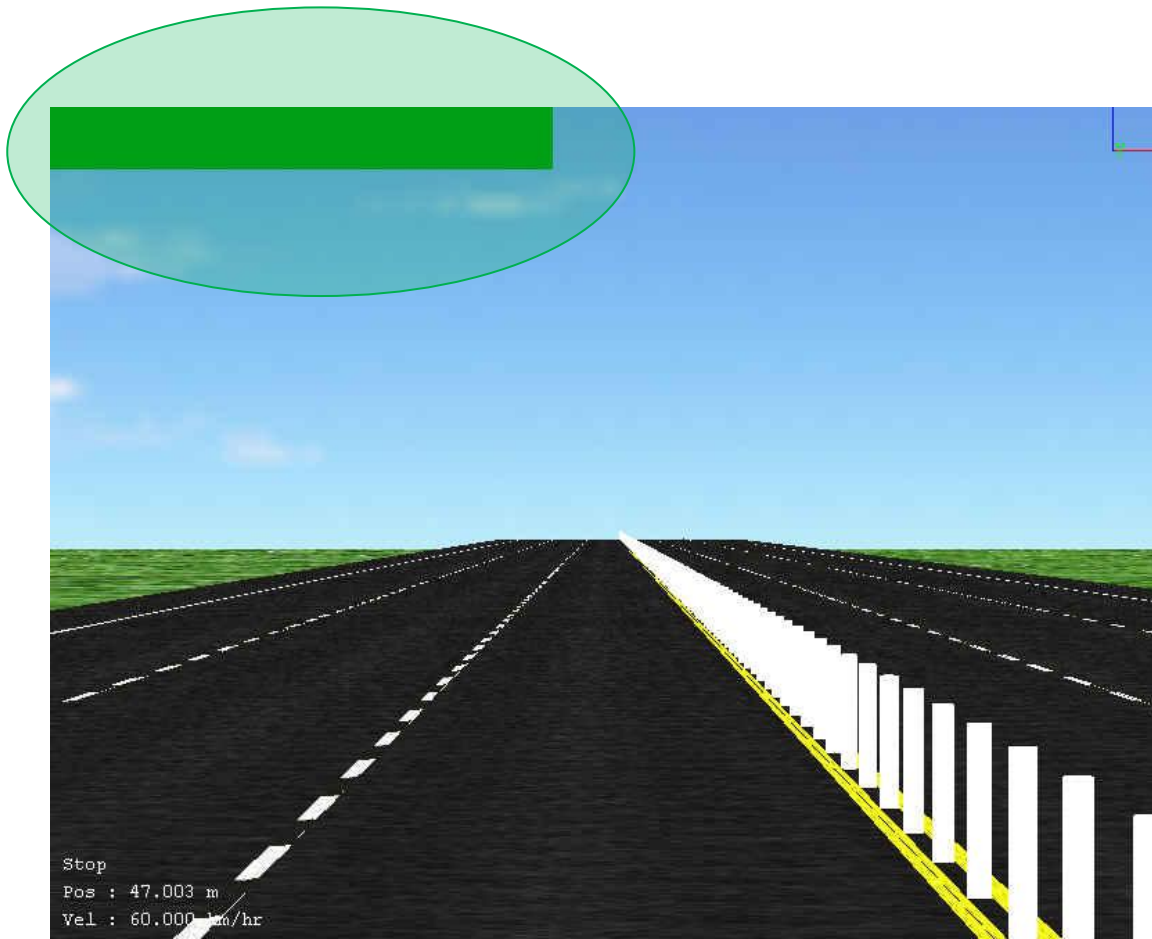
รูปแสดงระยะสิ้นสุดของการมองเห็นป้าย Gantry ขณะยานพาหนะแล่นด้วยความเร็ว 60 กิโลเมตรต่อชั่วโมง บนทางหลวงชนบท 6 ช่องจราจร
