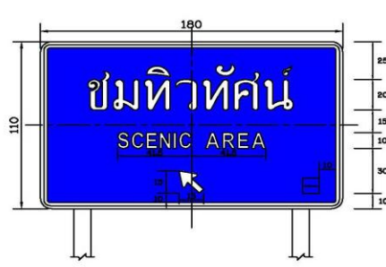
ป้ายแสดงสถานที่ชมทิวทัศน์
