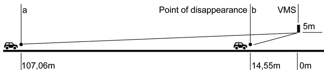
รูปแสดงหลักการมองเห็นป้าย VMS (Viewing distances and point of disappearance)
