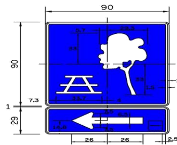
ป้ายแสดงที่พักริมทาง
